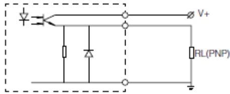
PNP 接线方式
